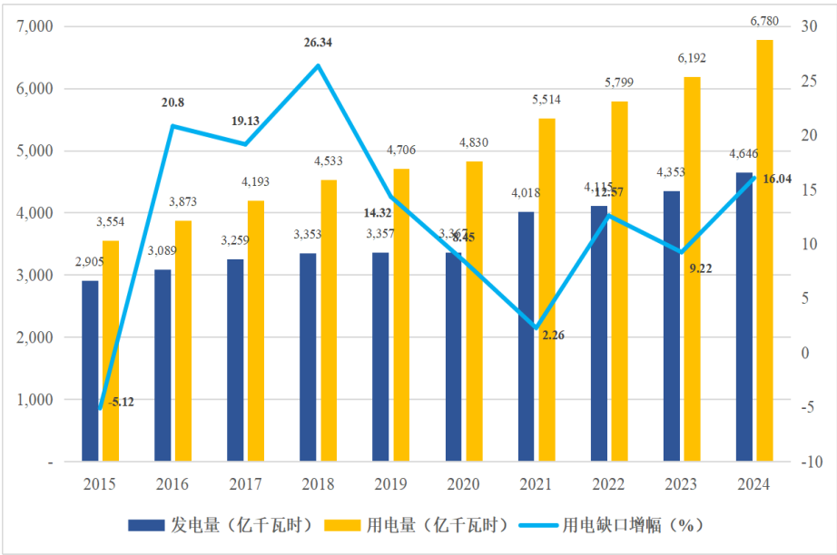
2015-2024 年浙江省发电量及用电缺口情况
