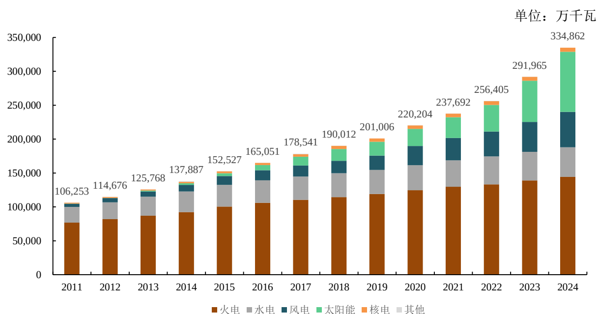
2011 年至 2024 年我国各类型发电装机容量情况
