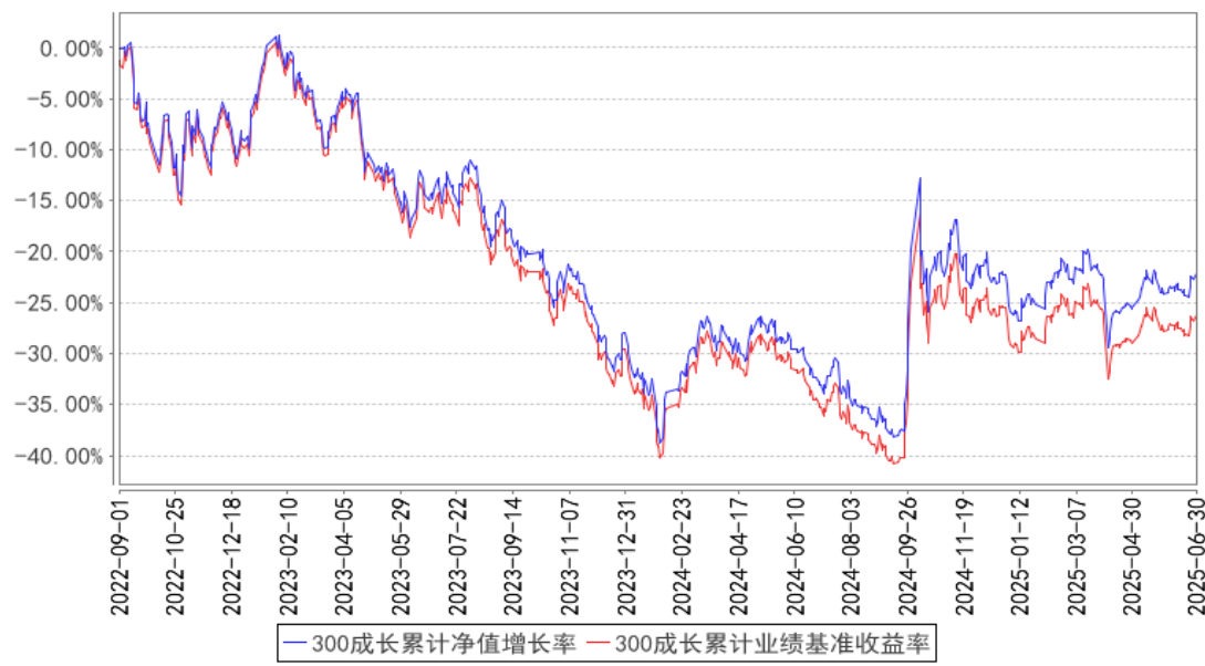
300成长累计净值增长率与同期业绩比较基准收益率的历史走势对比图
