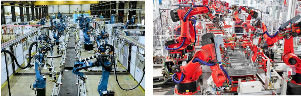
图 4. 新能源汽车焊装自动化生产线
