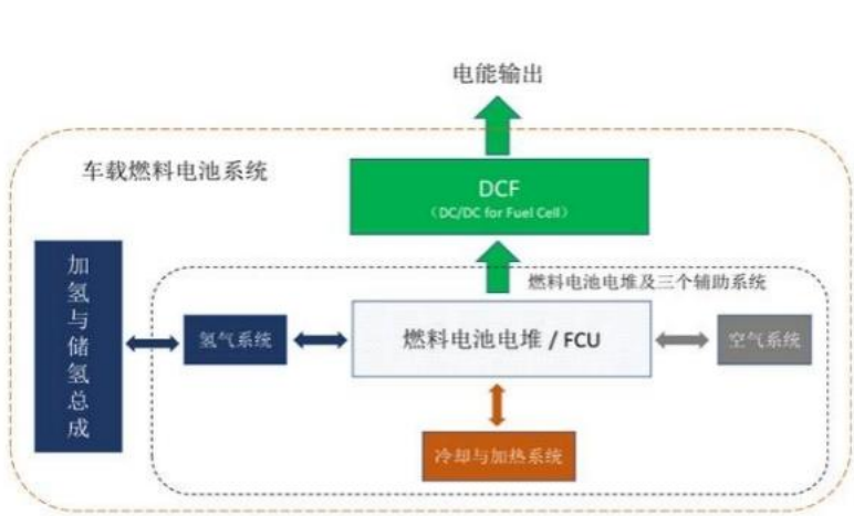
燃料电池系统的拓扑结构
