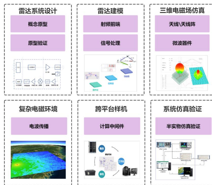
图 7：公司半实物仿真系统原理图
