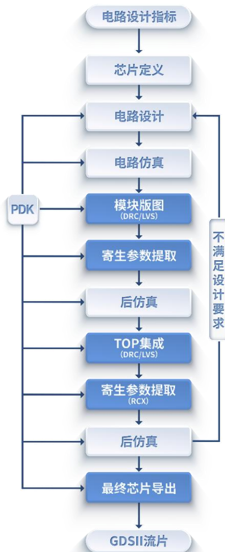
图 6：蓝色方框步骤为芯片版图设计步骤
