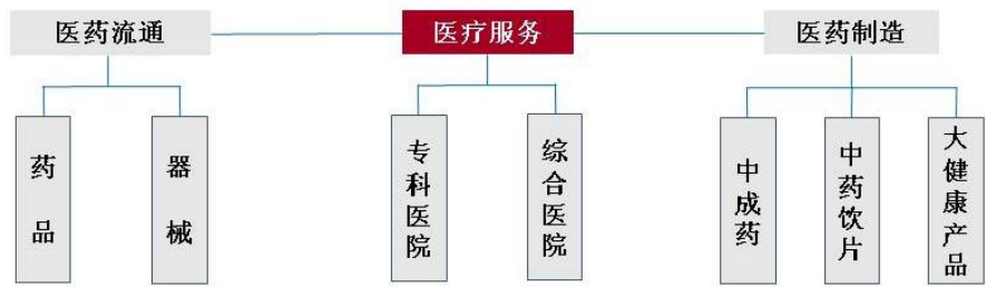
业务架构
