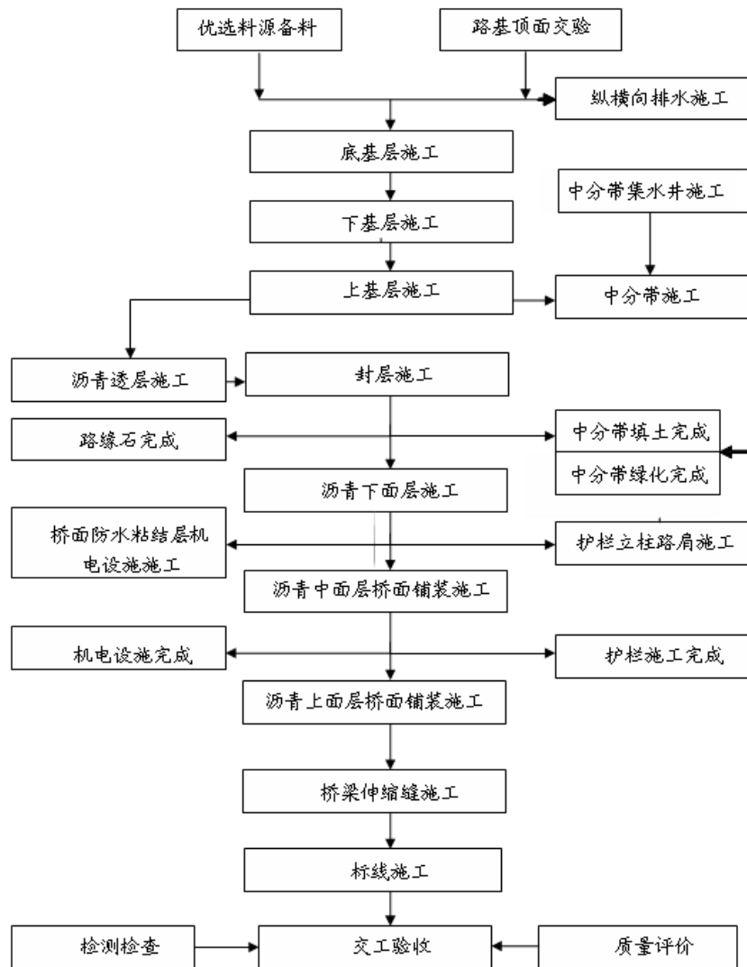
桥梁、桥涵工程施工工艺流程图
