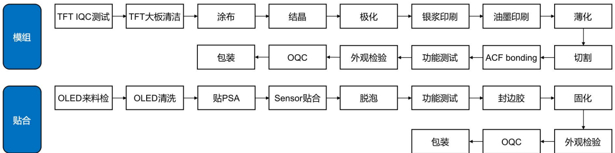
(3) 超声波指纹识别模组工艺流程图
