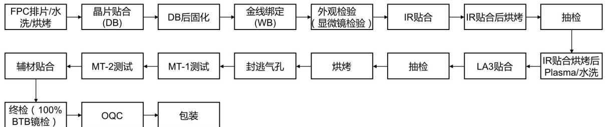
(3) 超声波指纹识别模组工艺流程图
