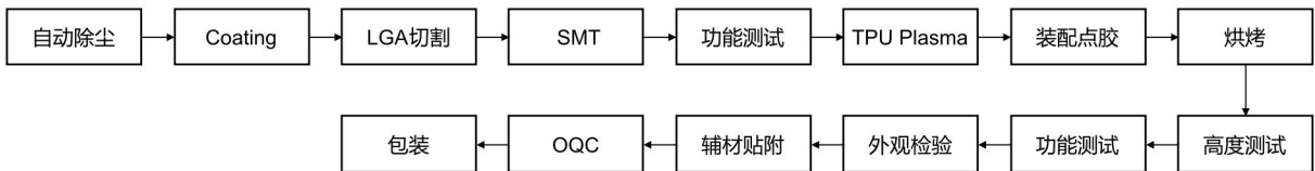
(2) 光学式屏下指纹识别模组工艺流程图
