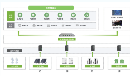
拓邦零碳云——云边端架构图
