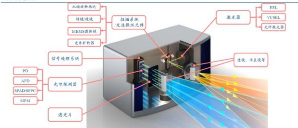
激光雷达构成
