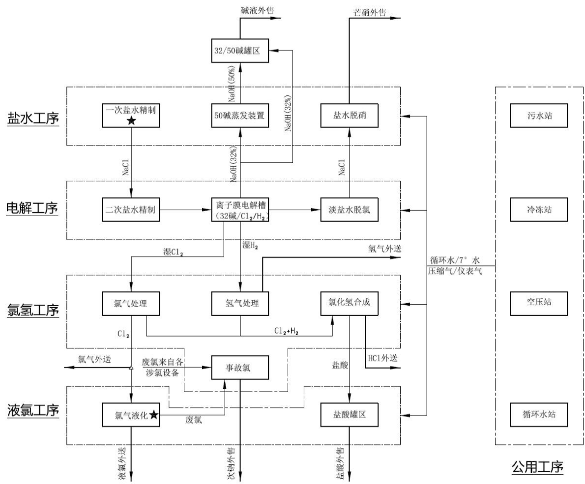
三门峡铝业烧碱生产工艺流程图
