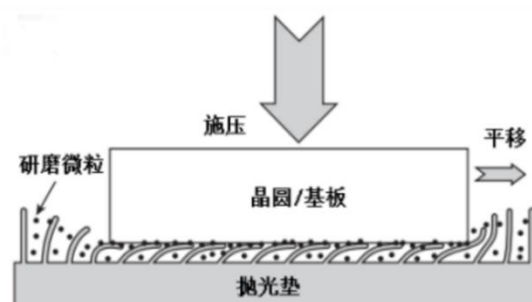
CMP抛光作业原理图
