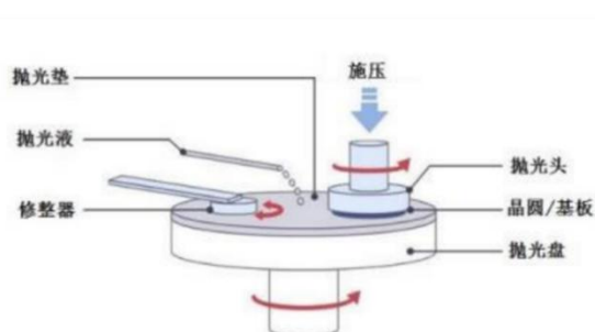
CMP抛光模块示意图
