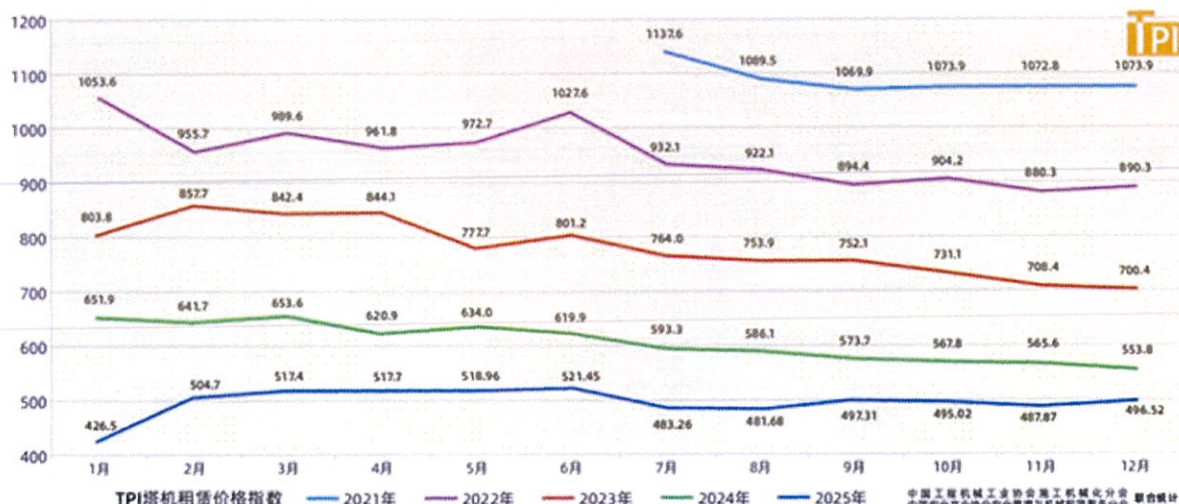
行业协会联合统计的塔机租赁价格指数
