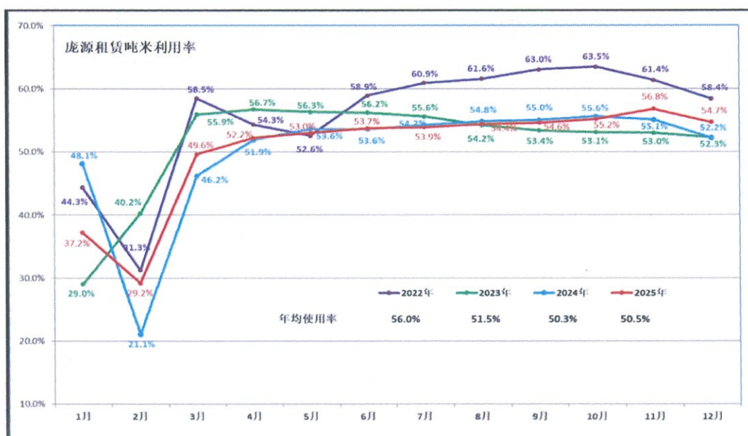
庞源在线统计的塔机吨米利用率数据
