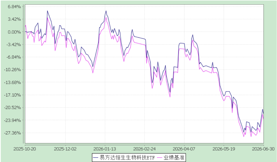
易方达恒生生物科技交易型开放式指数证券投资基金 累计净值增长率与业绩比较基准收益率的历史走势对比图 (2025 年 10 月 20 日至 2026 年 6 月 30 日)
