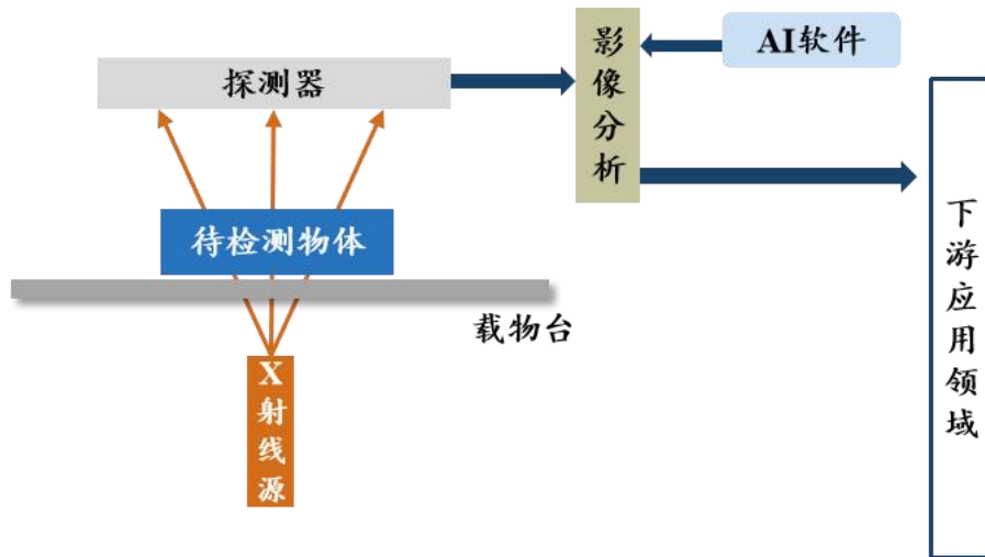
图一：X 射线检测设备原理图解
