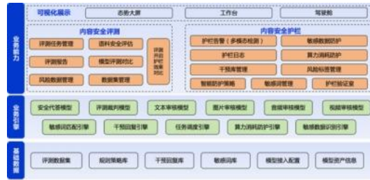
360 大模型卫士内容安全评测与内容安全护栏两大模块
