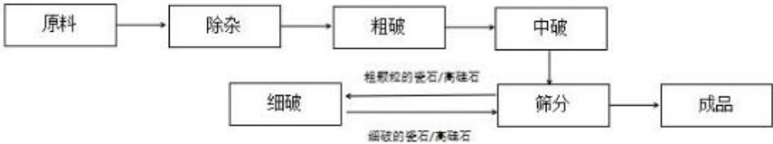
破碎车间生产工艺流程图
