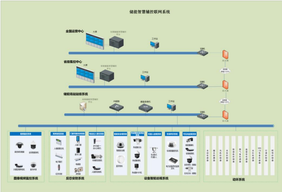
图：储能电站智能辅控系统解决方案
