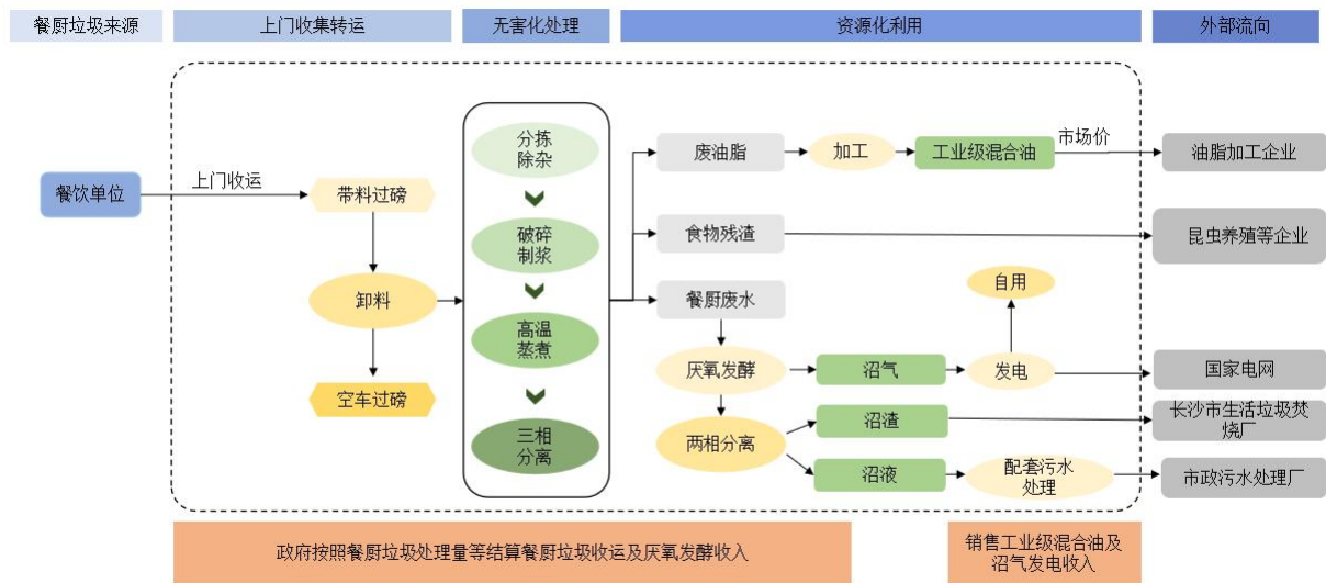
图 7 公司餐厨垃圾处理项目工艺示意图
