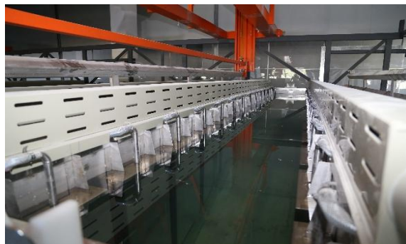
龙门挂镀镍产线
