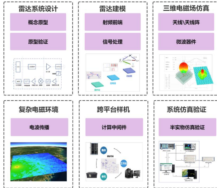
图 5：公司半实物仿真系统原理图
