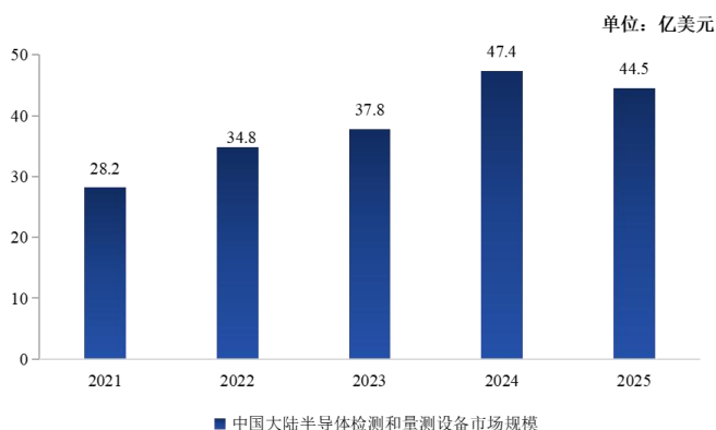
2021-2025年 中国大陆半导体检测和量测设备市场规模及增速情况
