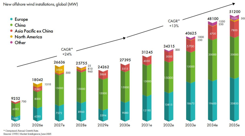
图：2025-2035 年全球海上风电装机预测，来源：全球风能理事会
