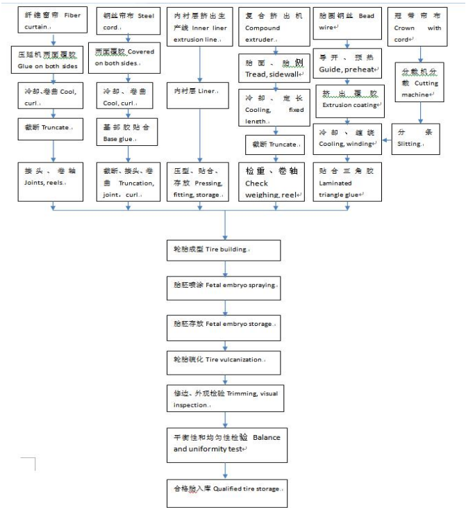
生产工艺流程图
