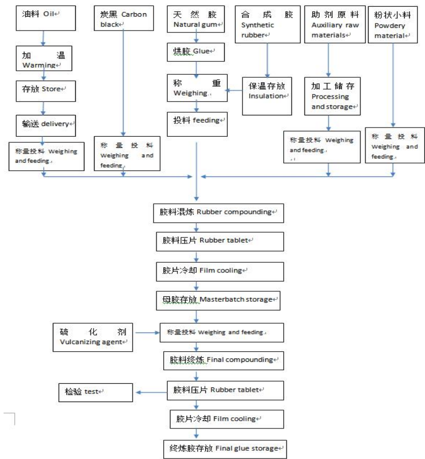
工艺流程图 胶料制造工艺流程图
