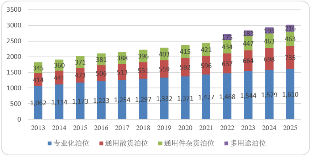
2013-2025 年全国万吨级及以上码头泊位构成情况（单位：个）
