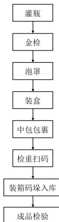
包装工艺流程图
