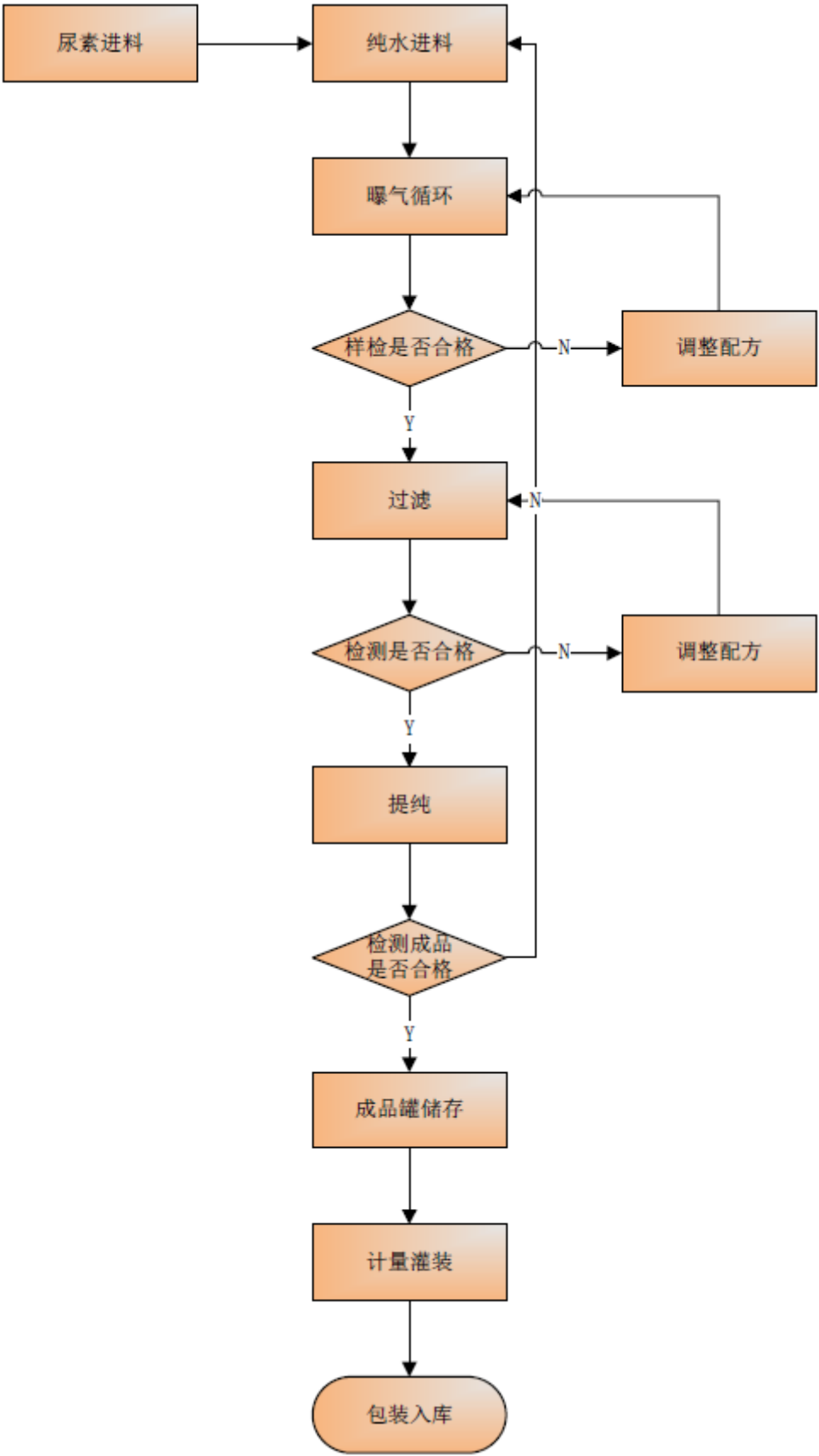
II 车用尿素溶液产品工艺流程图
