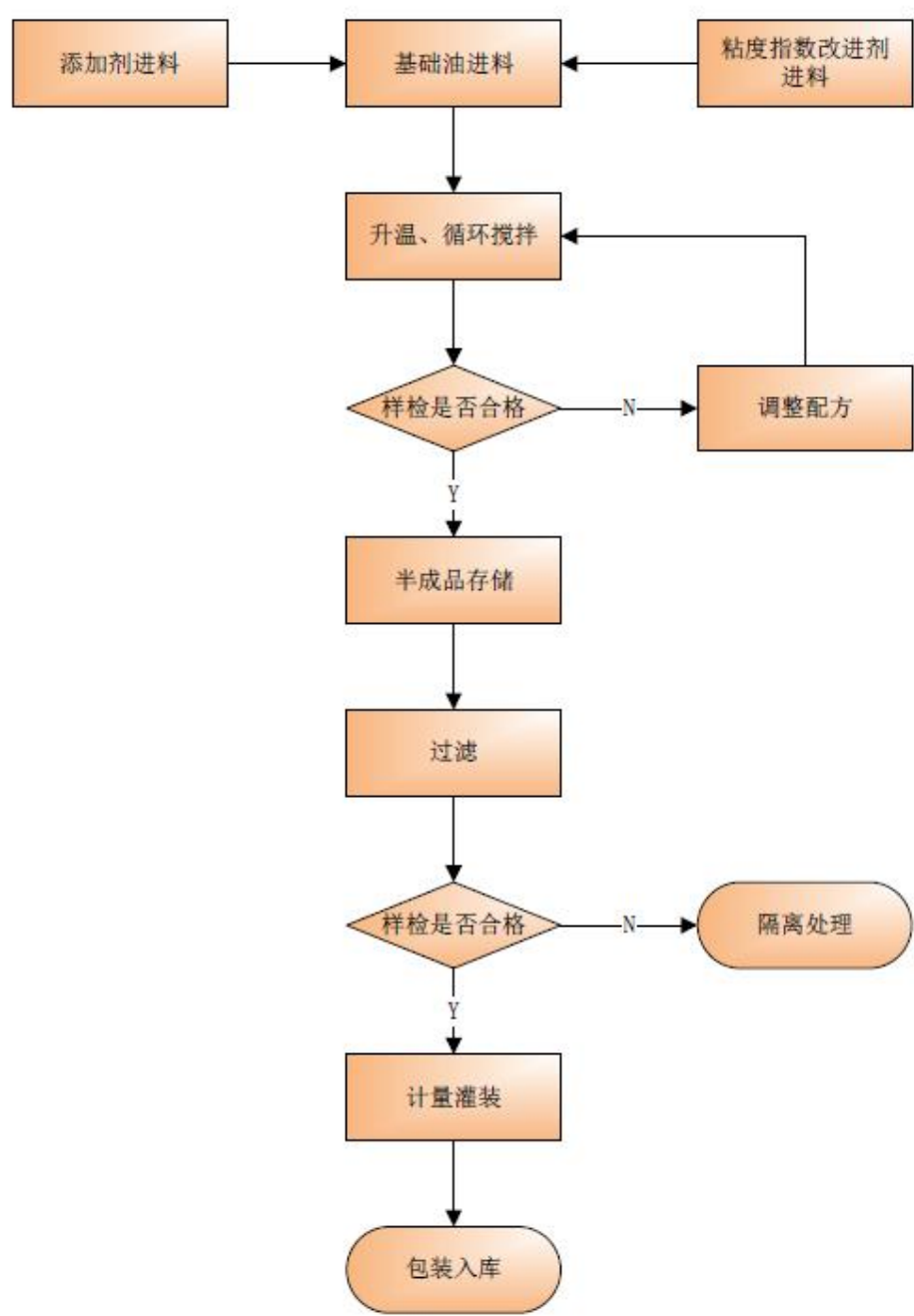
III 润滑油产品工艺流程图
