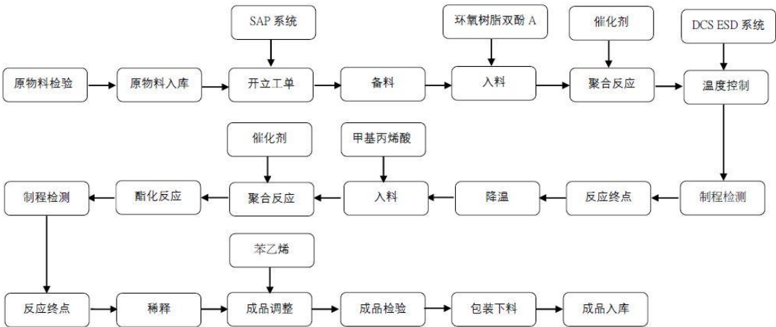
环保高性能耐腐蚀材料工艺流程图
