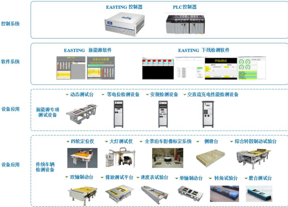
现代燃油汽车检测系统及解决方案中所包含主要测试设备如下：
