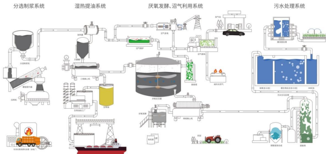
图 3：公司餐厨垃圾处置工艺流程图
