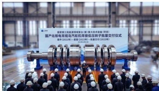
国产化核电常规岛汽轮机焊接低压转子批量交付
