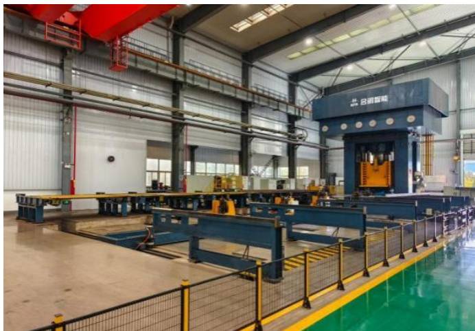
全自动道岔成型液压机生产线
