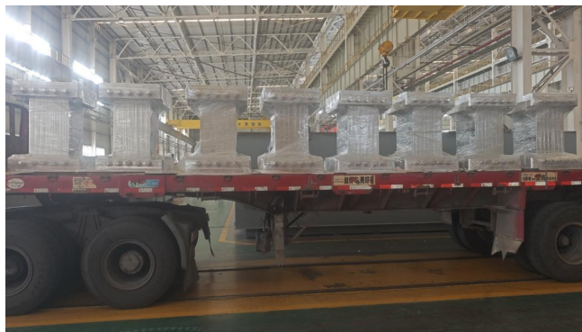
图3 重力支撑安装验收
