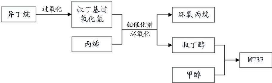
共氧化法环氧丙烷（PO/MTBE）生产工艺流程
