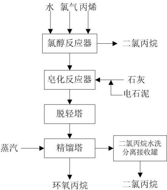
氯醇法环氧丙烷生产工艺流程
