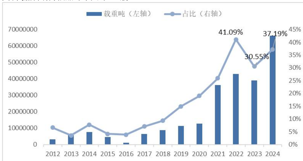
图 2. 替代燃料船舶订单量 and 在新船订单中的比重
