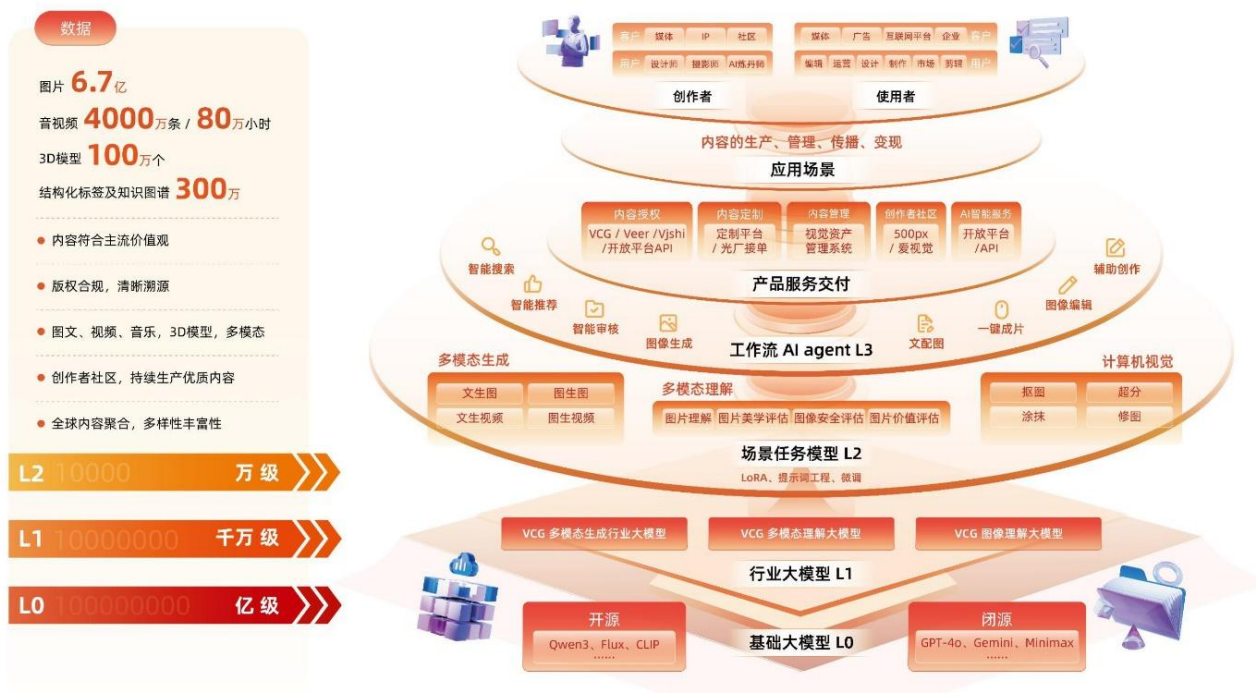
图示：基础大模型（L0）提供的是通用的模型能力，不针对任何特定使用场景；垂直领域或者行业领域大模型（L1）结合某个领域的通用知识或技能做了针对性的训练，但不针对某一个具体应用场景；场景任务模型，是在 L0 或 L1 任一种的基础上结合用户需求和和使用场景所做的极具针对性的训练形成的模型，结合 AI 智能体与 workflow，用于解决具体问题，提供直接满足用户需求的方案和结果。
