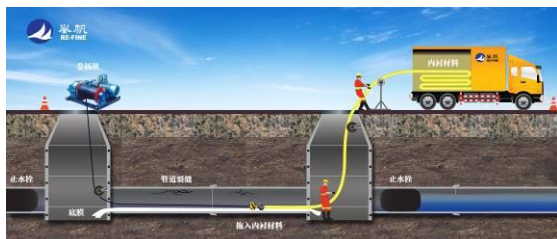
拖入底膜，拉入内衬材
