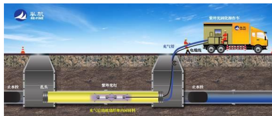
鼓风吹气，送入紫外灯架，紫外固化
