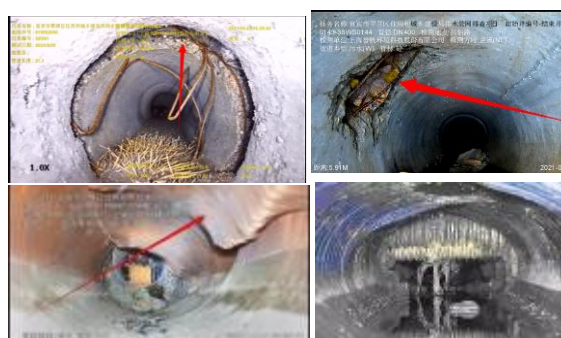
宜宾翠屏区结构性缺陷图
