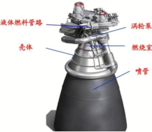
典型火箭发动机结构图
