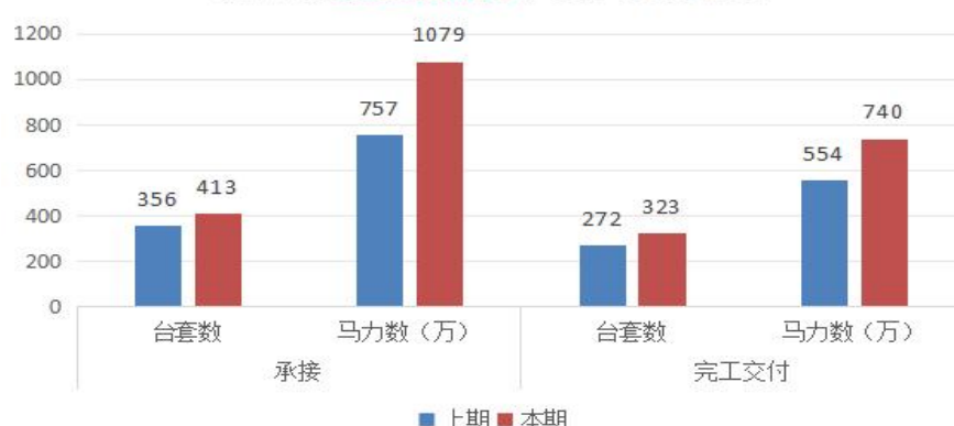
报告期低速柴油机承接和交付情况
