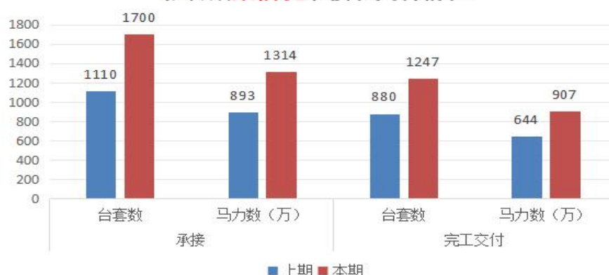
报告期柴油机承接和交付情况
