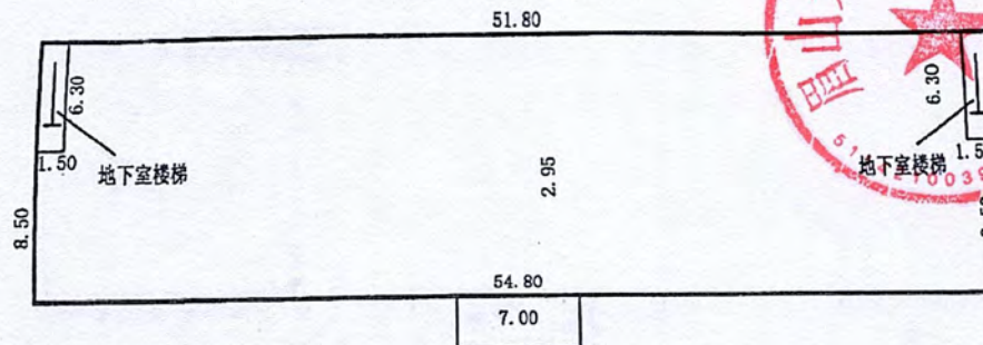
办公生活区A区(办公楼)1层平面图
